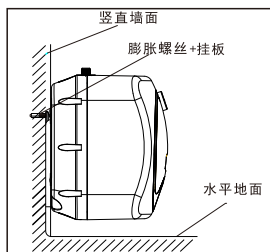
安装示意图 2
