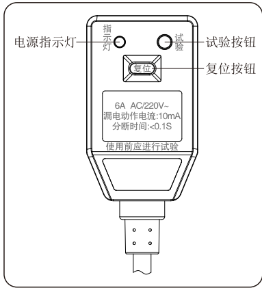
漏电保护插头部件位置示意图
