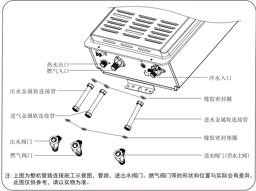
六、整机管路连接施工示意图
